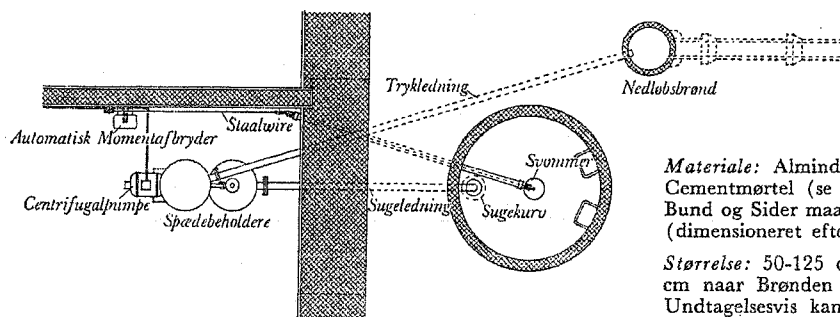
Pumpebrønd, Maal 1:50
